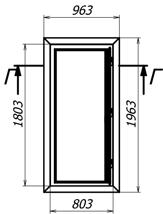
Г-Г (1 : 20)
