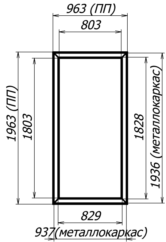
Д-Д (1 : 30) (Дверь не указана)
